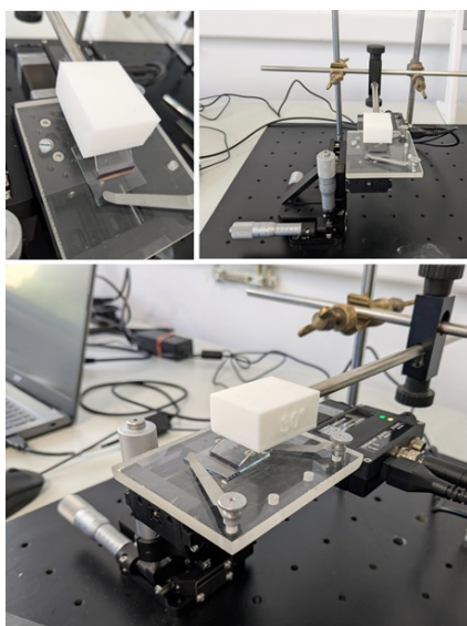
Dispozitiv Blade-coating
